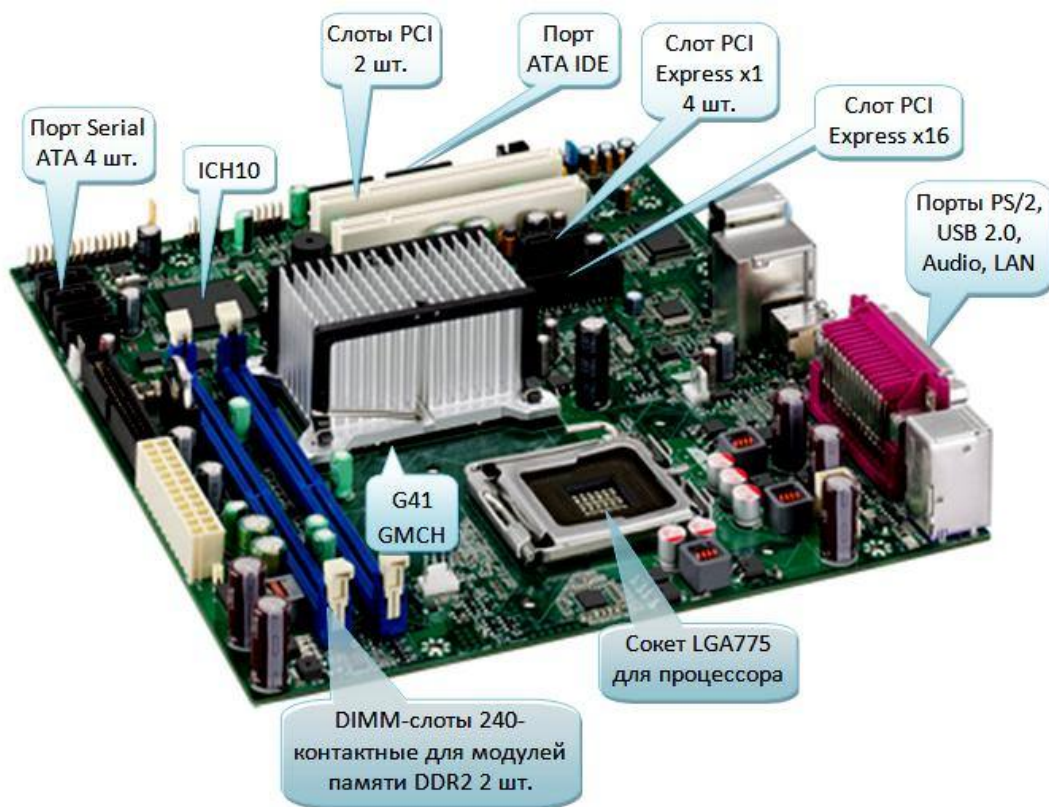
Рисунок 2.11. Материнская плата Intel DG41TY
