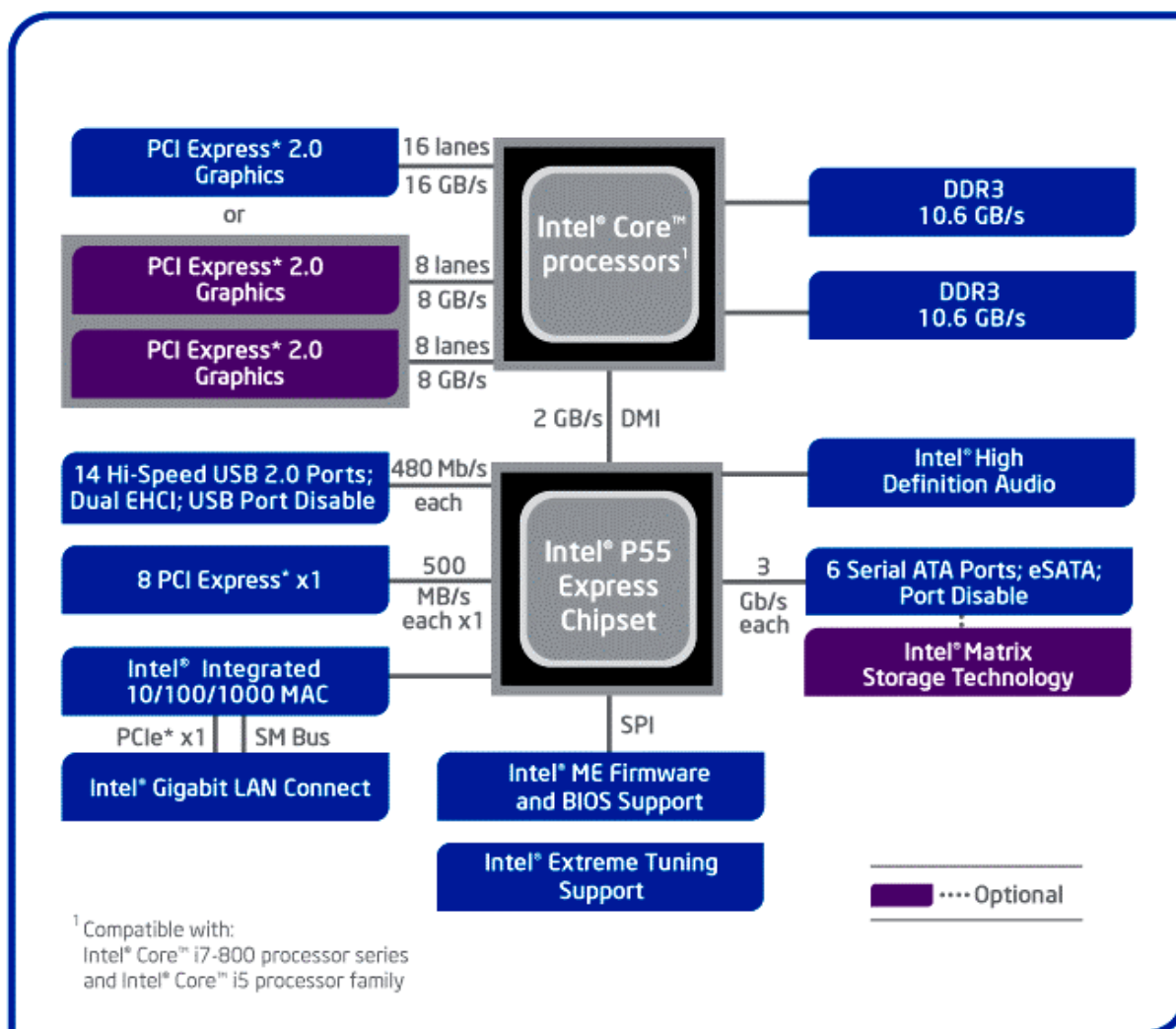
Рисунок 2.8. Блок-схема чипсета Intel® P55 Express
