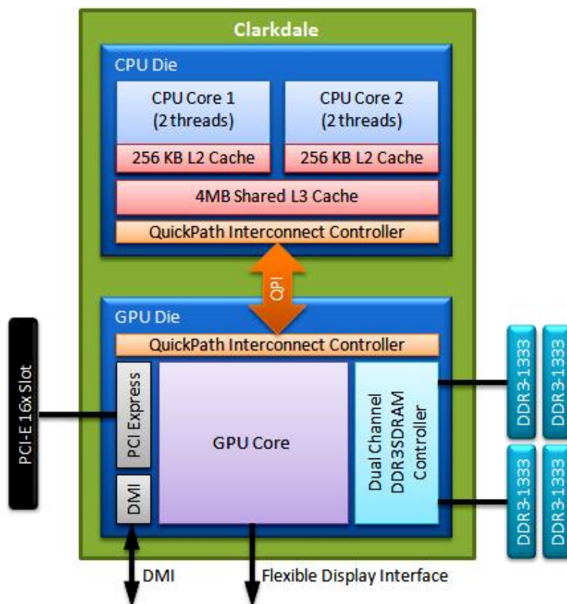
Рисунок 2.6. Блок-схема процессоров семейства Clarkdale
