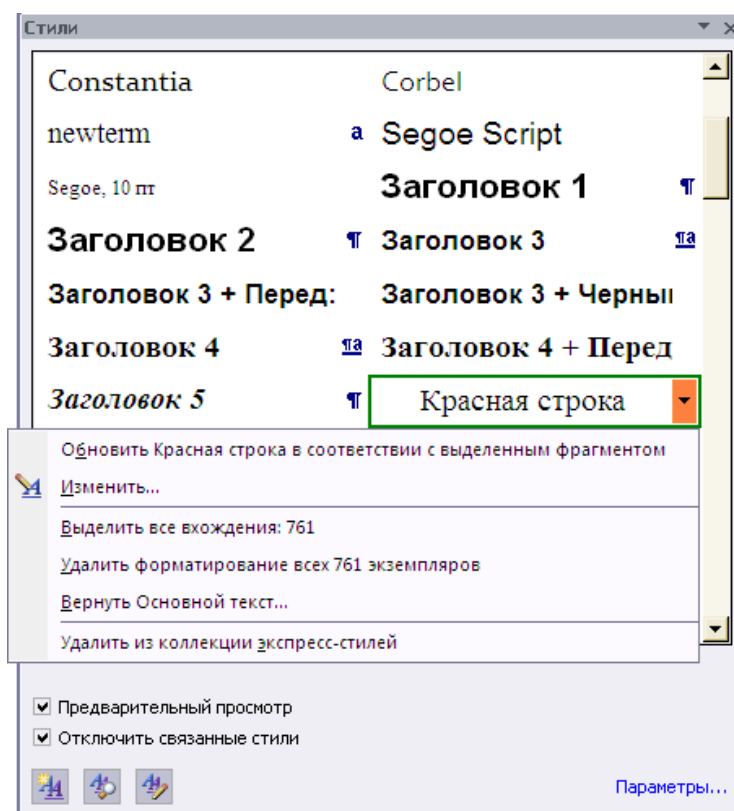
Рисунок 3.39. Окно «Стили»
