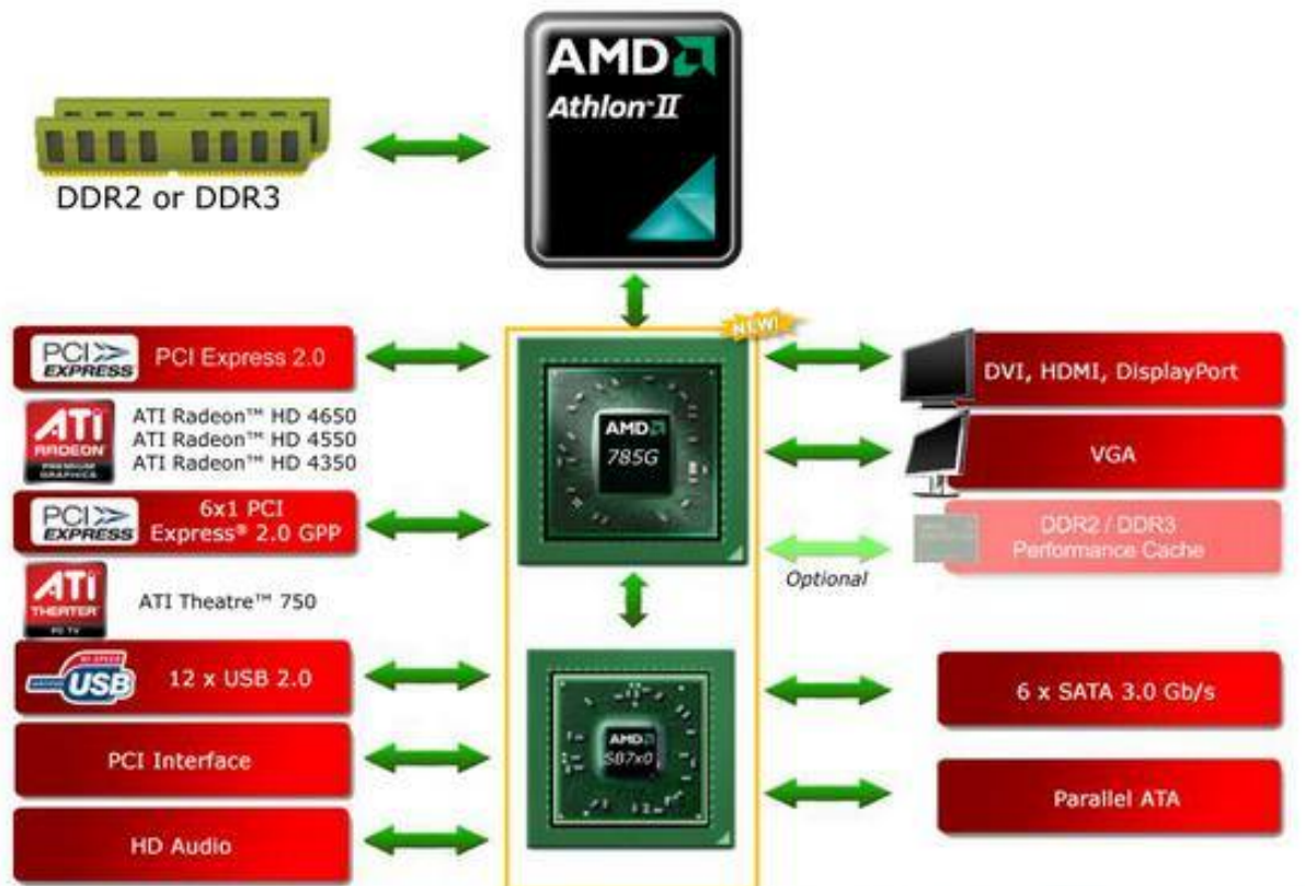
Рисунок 2.9. Чипсет AMD 780G
