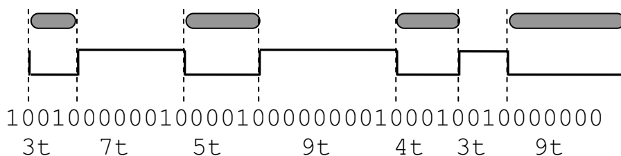
Рисунок 2.17. Схема преобразования при считывании информации с CD
