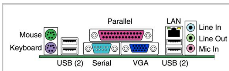
Рисунок 2.10. Пример портов внешних устройств на задней панели
