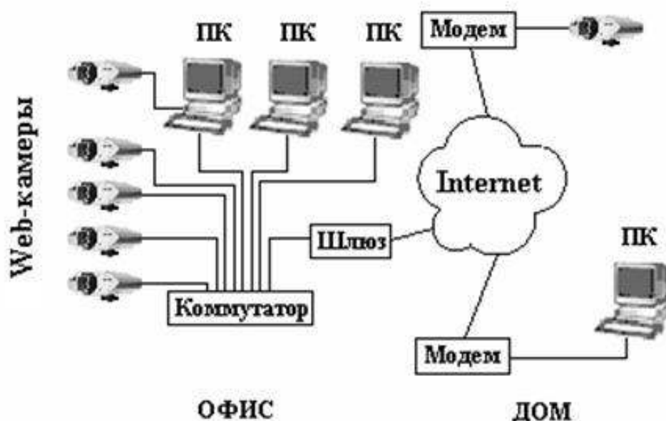
Рисунок 2.29. Варианты подключения Web-камер
