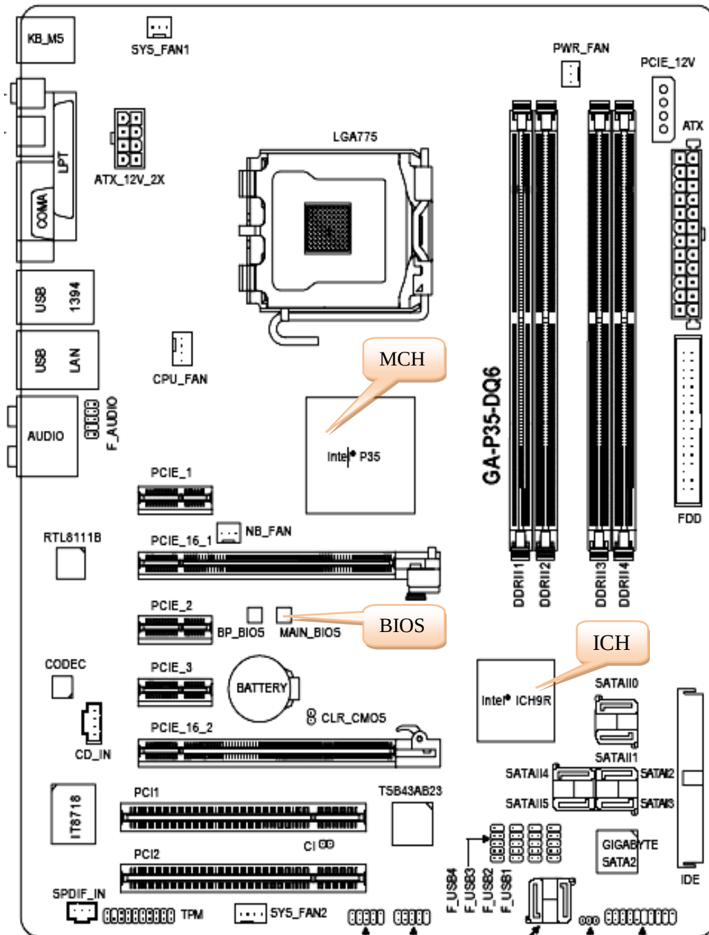
Рисунок 2.12. Схема материнской платы Gigabyte P35-DQ6
