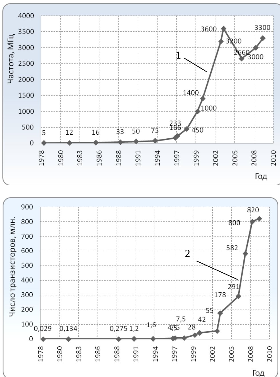
Рисунок 2.3. Графики изменения тактовой частоты (1) количества транзисторов (2) в процессорах фирмы Intel
