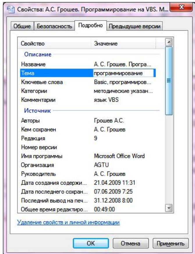
Рисунок 3.20. Свойства файла
