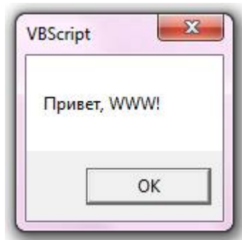
Рисунок 5.40. Простейший скрипт
